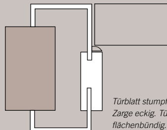
Türblatt stumpf einschlagend, Zarge flächenbündig, entsprechendes Wandöffnungsmaß muss bereits bei der Planung berücksichtigt werden.
