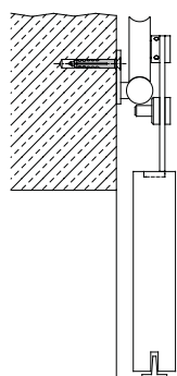
ART Montage Holztür ohne DUFU
