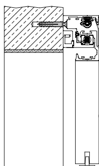
MOVE Montage Holztür ohne DUFU mit Distanzprofil
