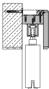
KLASSIK Montage Holztür ohne DUFU
