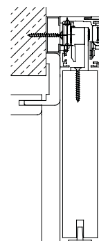
SLIM Montage Holztür mit DUFU und Distanzprofil
