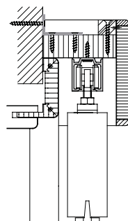
KLASSIK Montage Holztür mit DUFU
